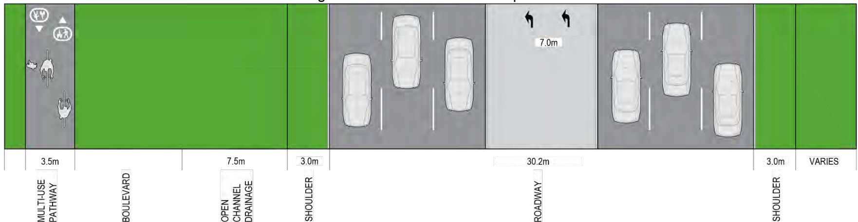
PLAN Lagamodière Boulevard - Concept-1B & 2B
